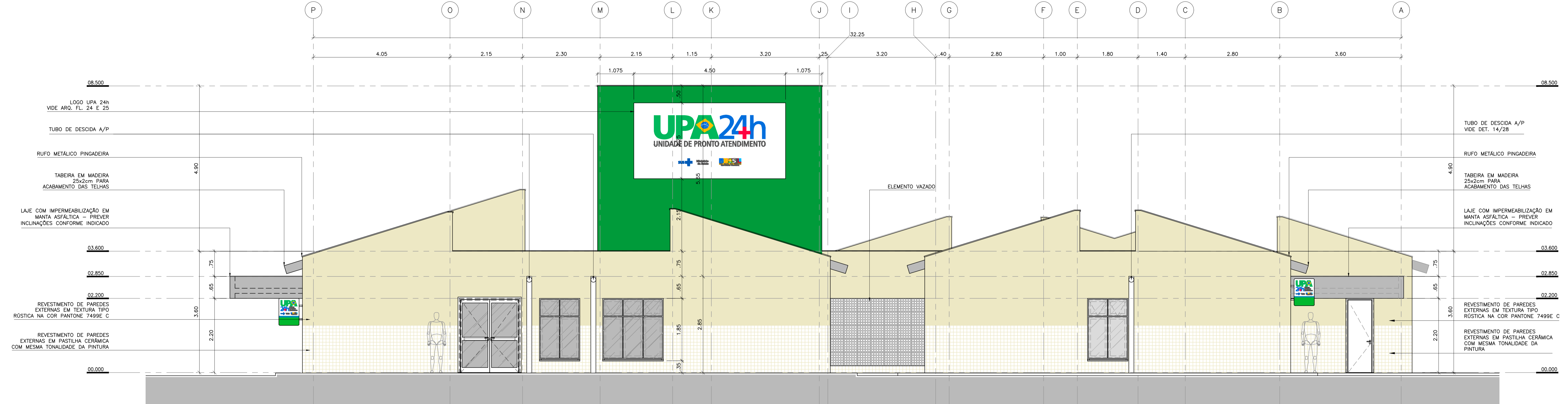
02 UNIDADE DE PRONTO ATENDIMENTO – PORTE 2 FACHADA 02 ESCALA: 1:50
